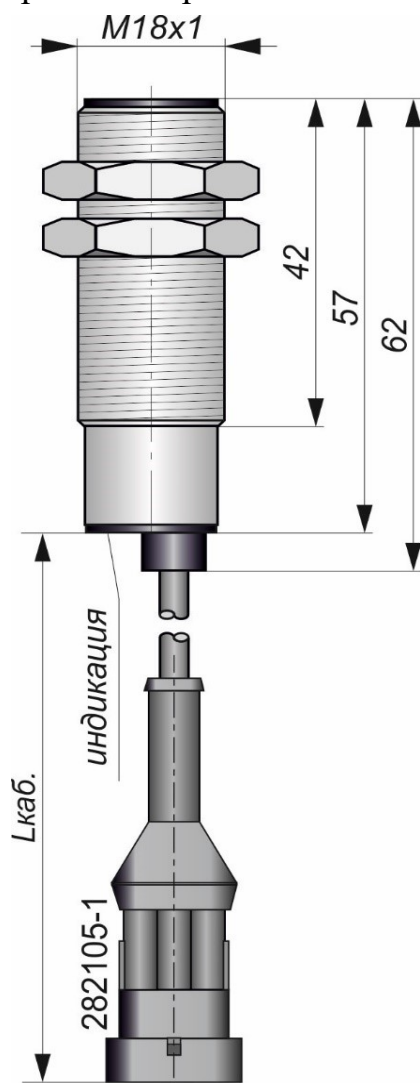
Габаритный чертеж
