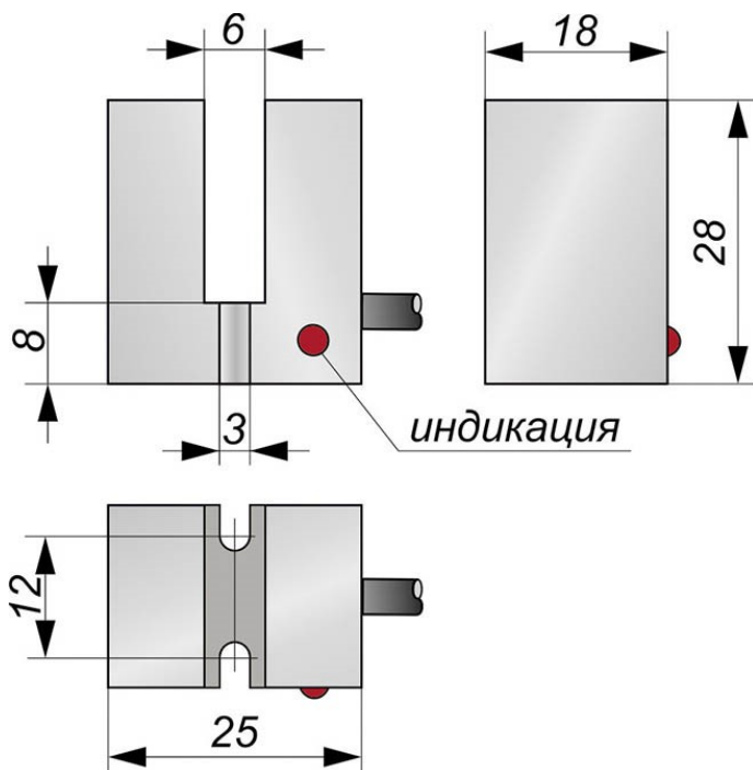
Габаритный чертеж
