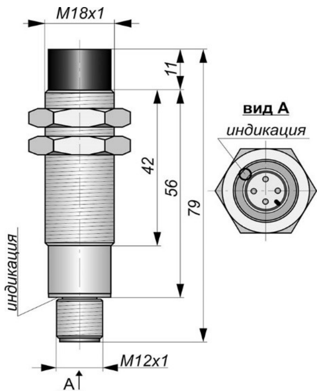
Габаритный чертеж
