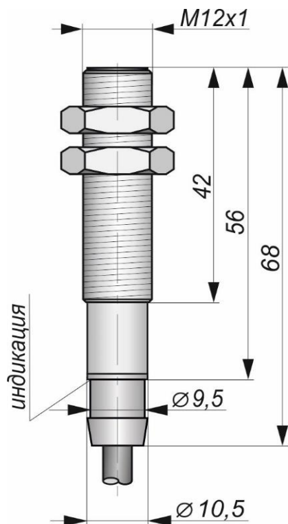
Габаритный чертеж
