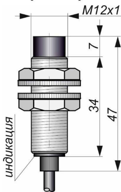
Габаритный чертеж
