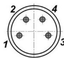
Цоколевка разъема
