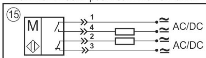
Гальванически-развязанные контакты
