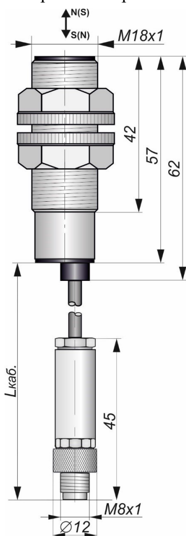
Габаритный чертеж
