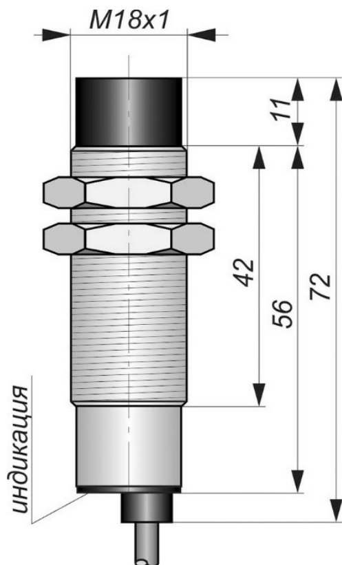
Габаритный чертеж
