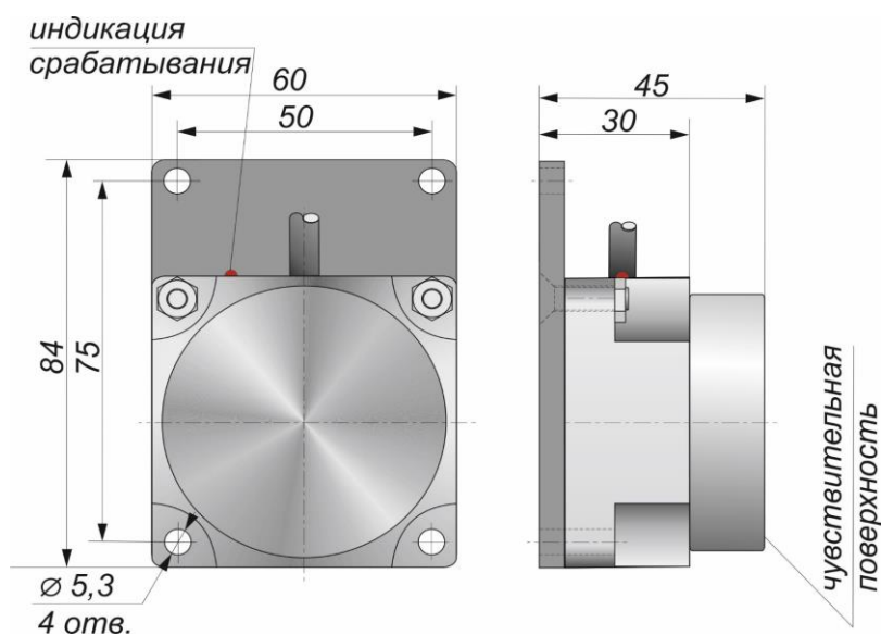
Габаритный чертеж
