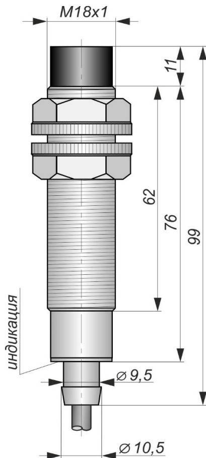
Габаритный чертеж
