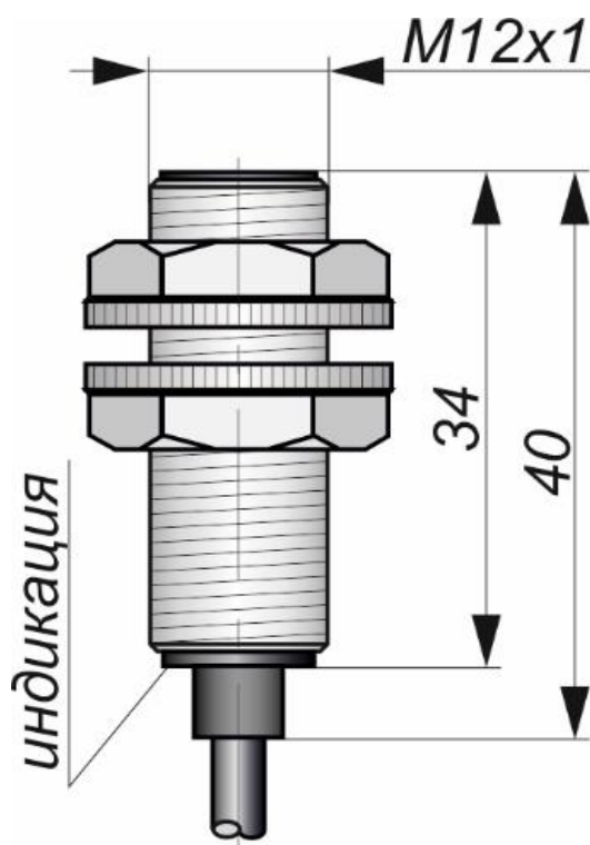
Габаритный чертеж
