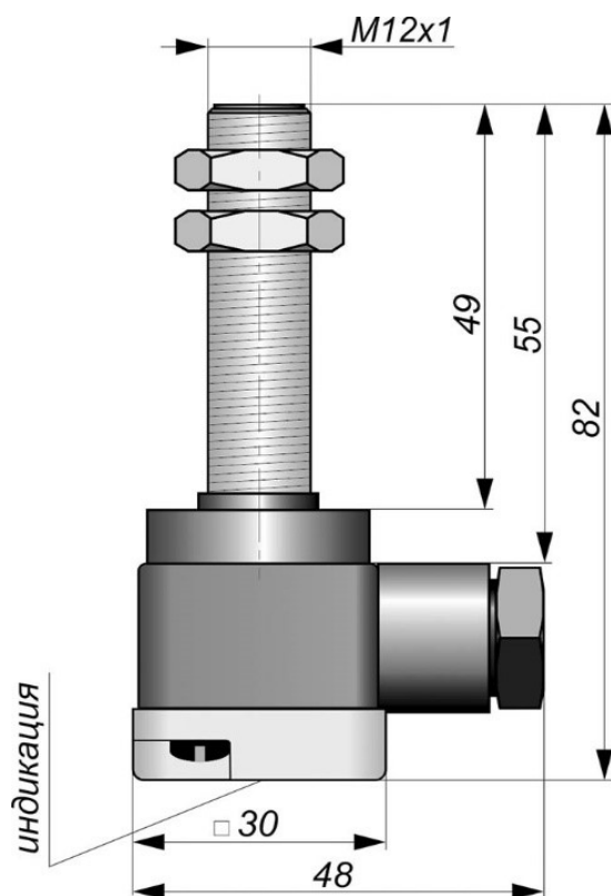
Габаритный чертеж
