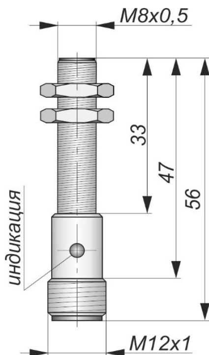
Габаритный чертеж
