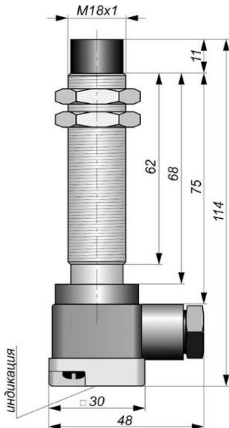
Габаритный чертеж
