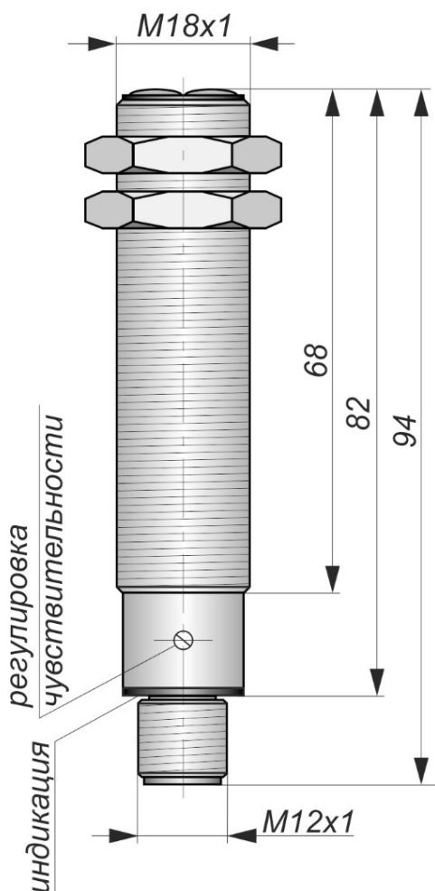
Габаритный чертеж
