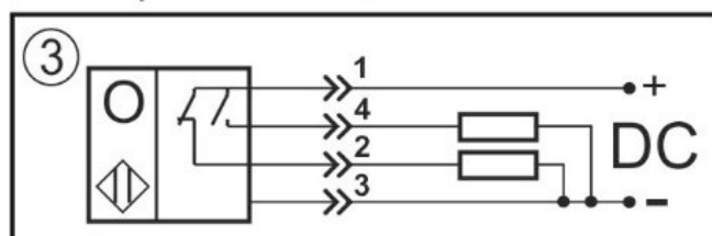
Переключающий контакт
