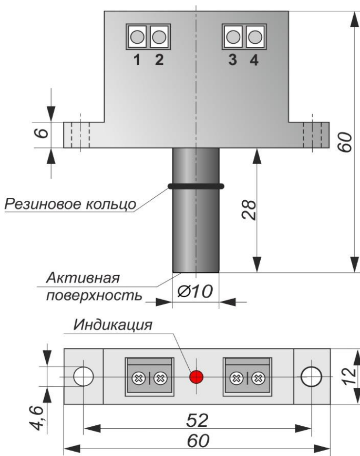
Габаритный чертеж
