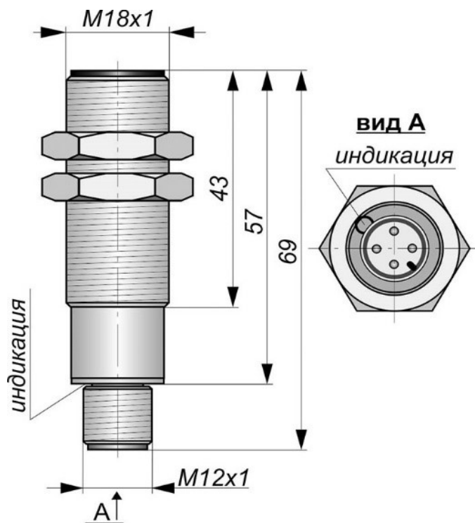
Габаритный чертеж
