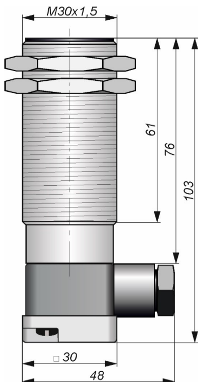
Габаритный чертеж
