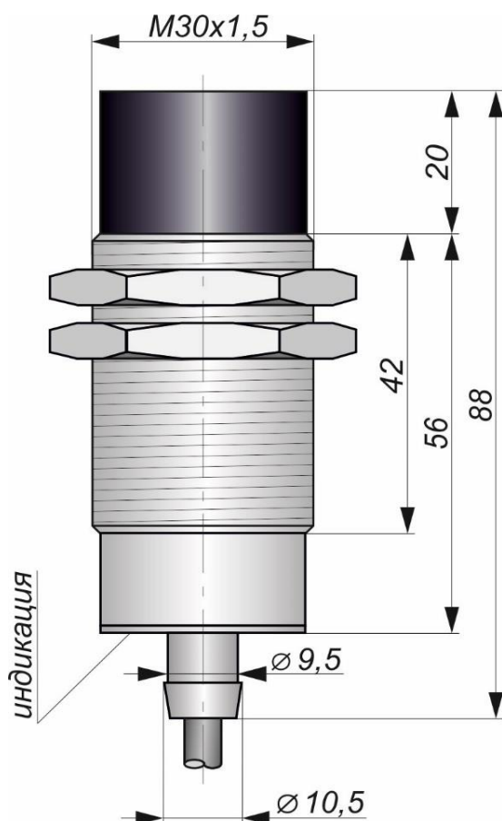
Габаритный чертеж
