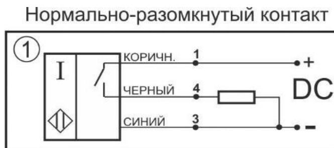
Схема соединения
