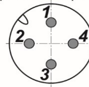
Цоколевка разъема
