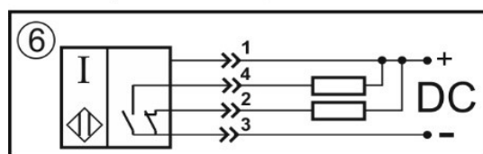
Переключающий контакт
