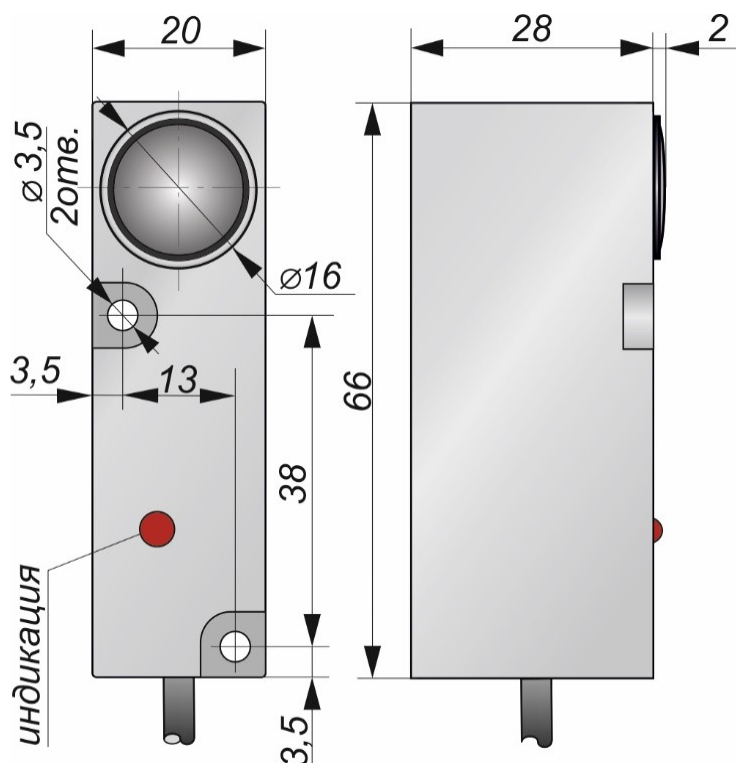
Габаритный чертеж
