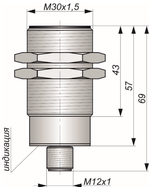
Габаритный чертеж
