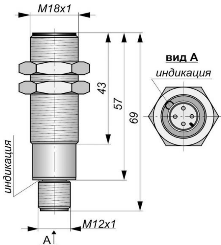
Габаритный чертеж
