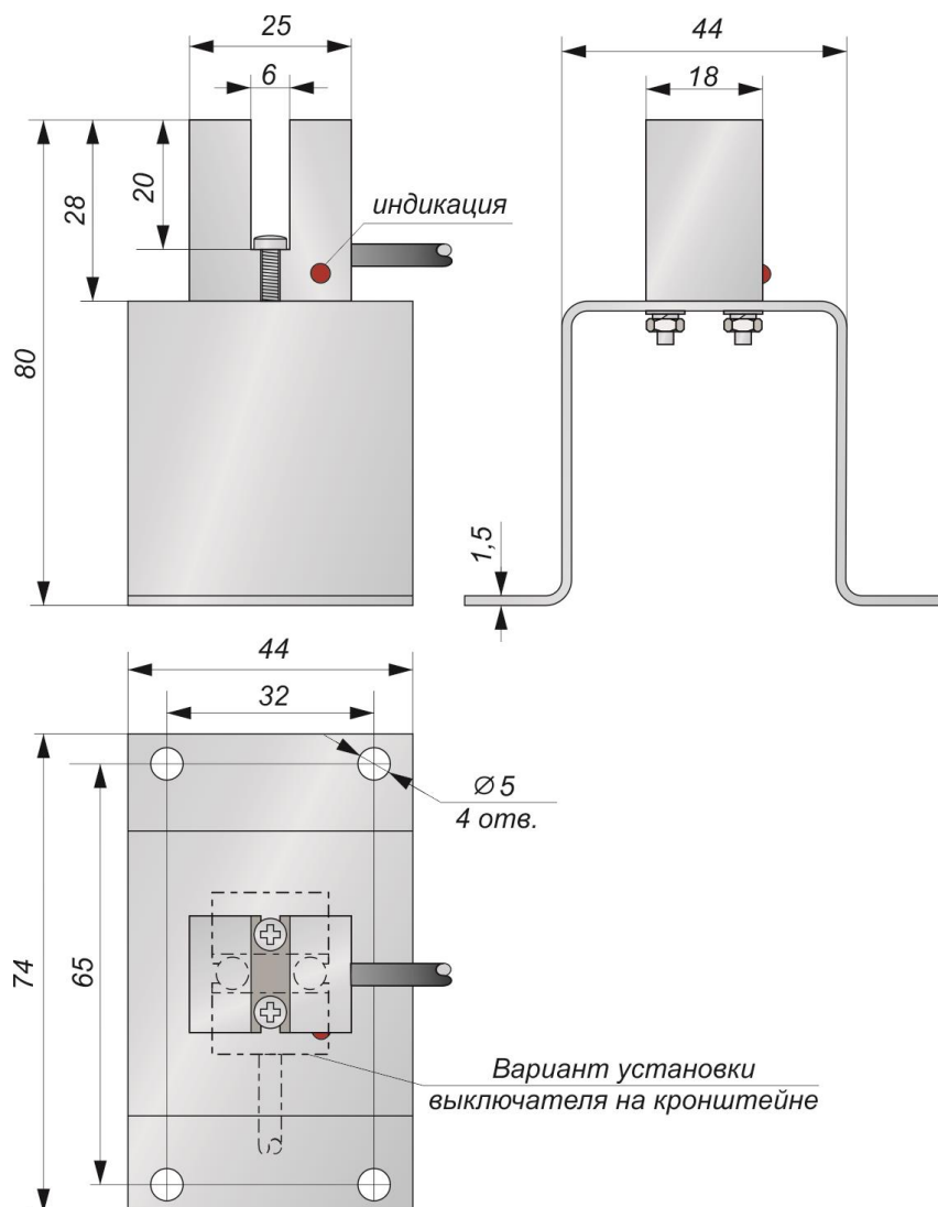
Габаритный чертеж
