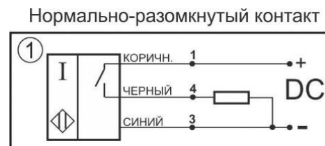
Схема соединения
