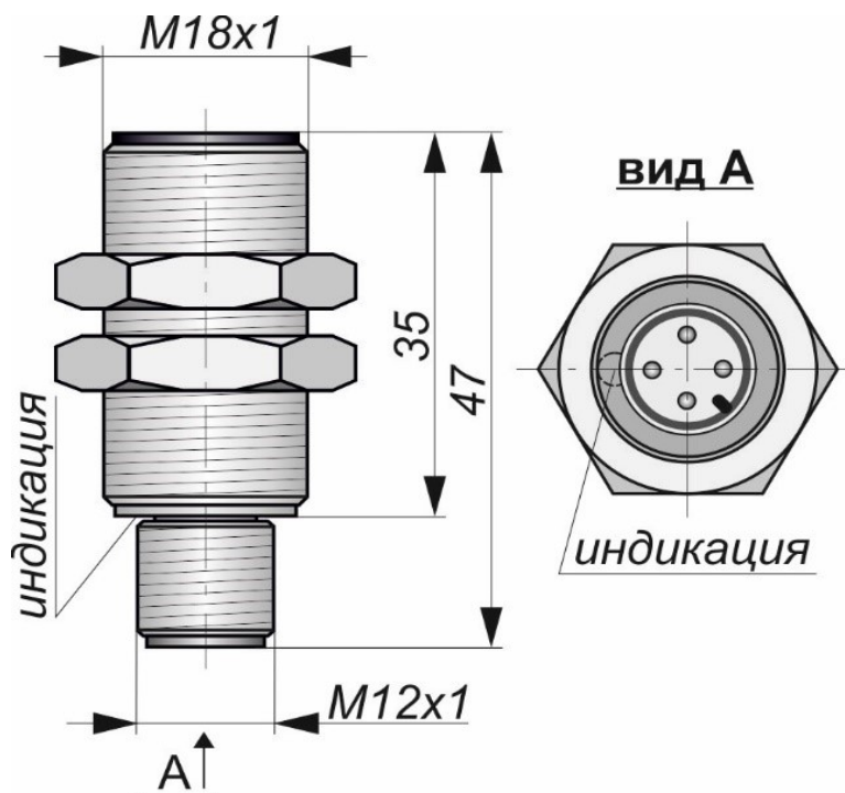
Габаритный чертеж
