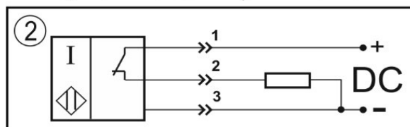
Цоколевка разъема
