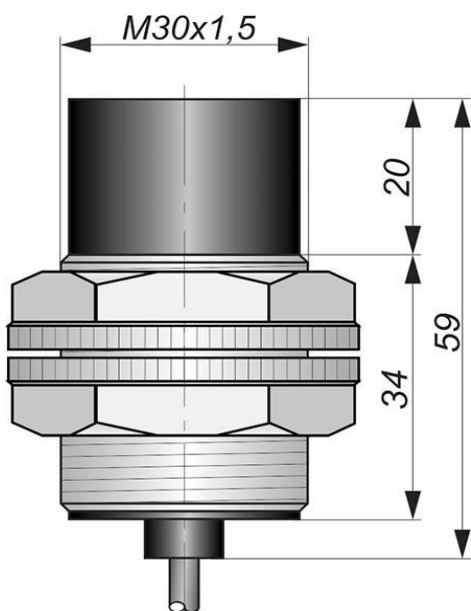
Габаритный чертеж
