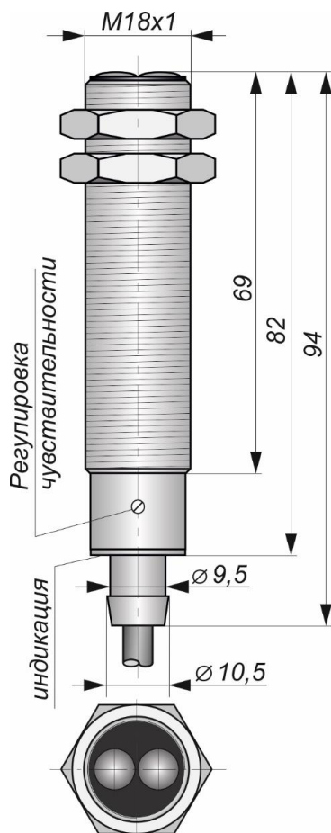
Габаритный чертеж
