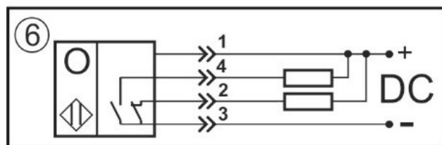
Переключающий контакт
