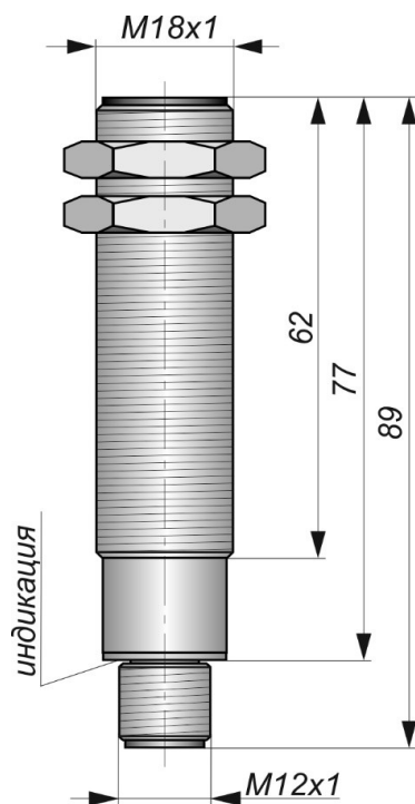
Габаритный чертеж
