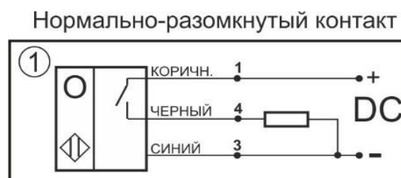
Схема соединения
