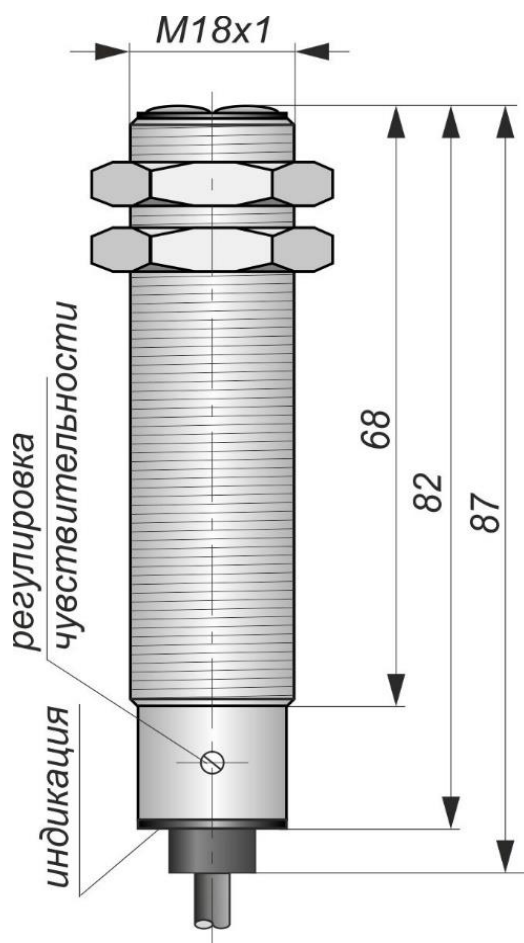
Габаритный чертеж
