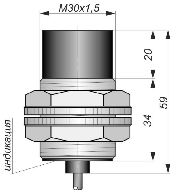
Габаритный чертеж
