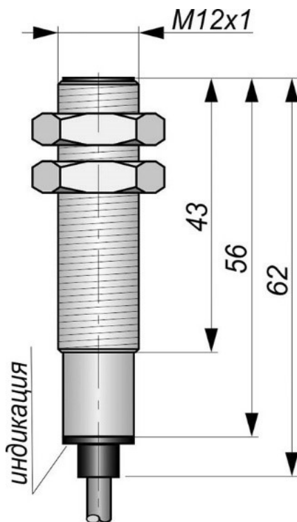
Габаритный чертеж
