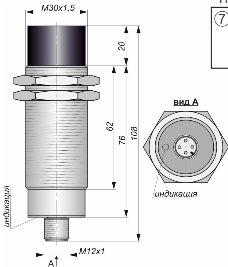
Габаритный чертеж
