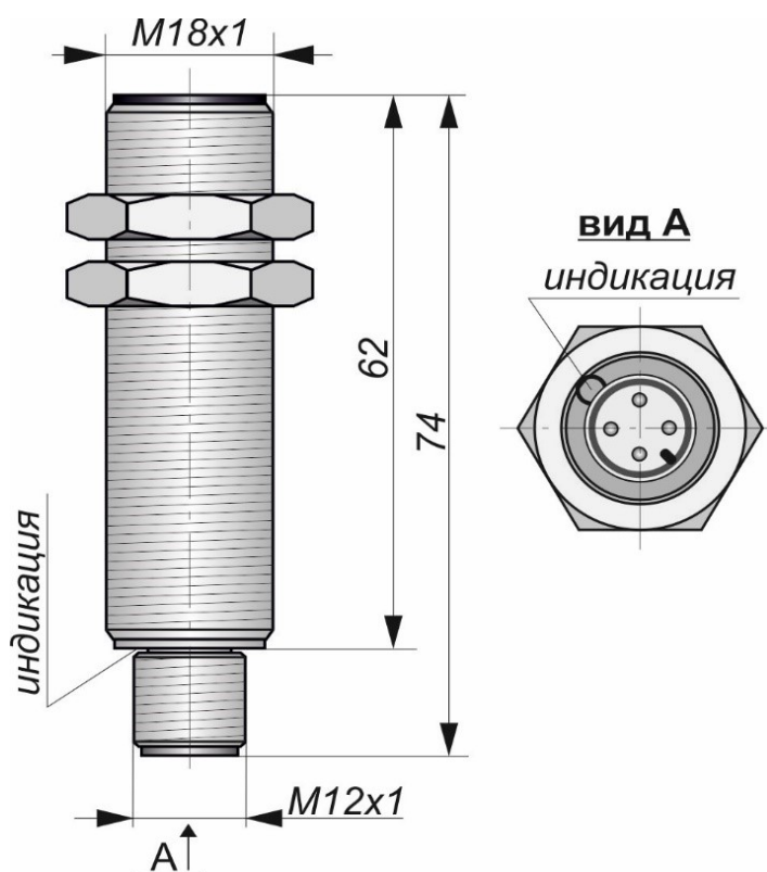
Габаритный чертеж
