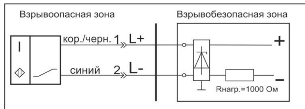
Схема соединения
