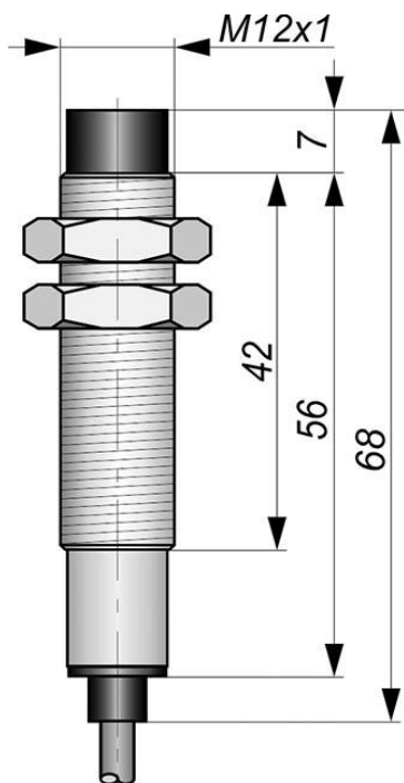
Габаритный чертеж
