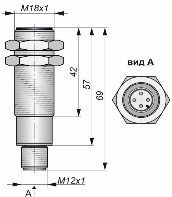
Габаритный чертеж
