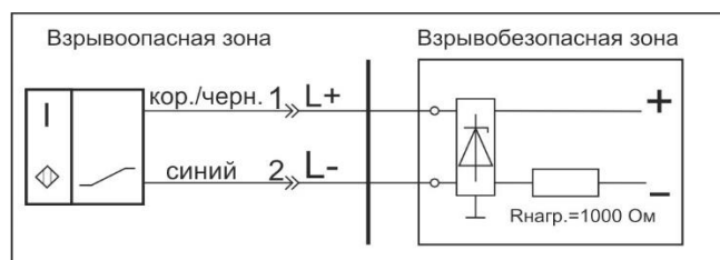
Цоколевка разъема
