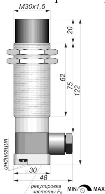
Габаритный чертеж
