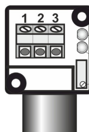
Цоколевка клеммной колодки
