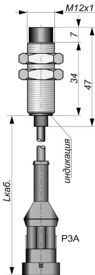
Габаритный чертеж
