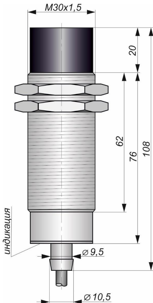
Габаритный чертеж
