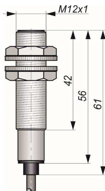
Габаритный чертеж
