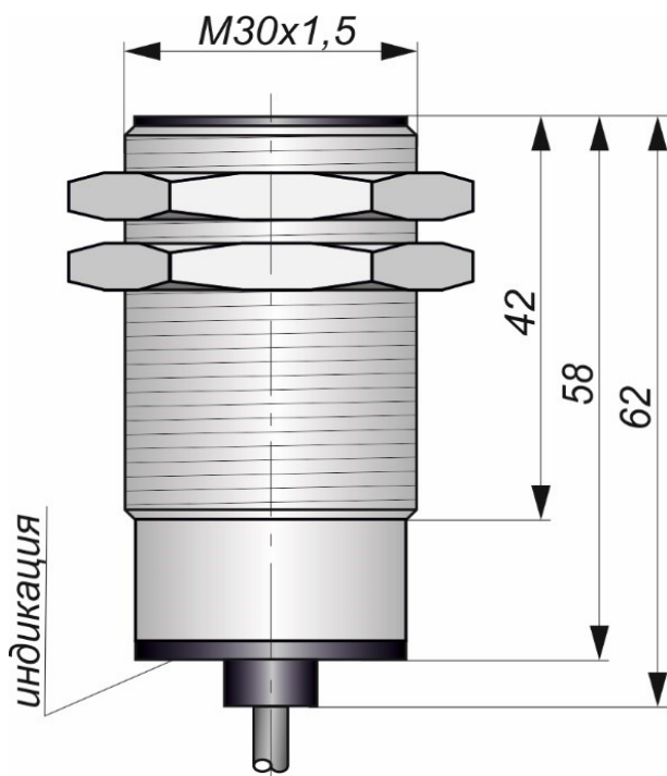
Габаритный чертеж
