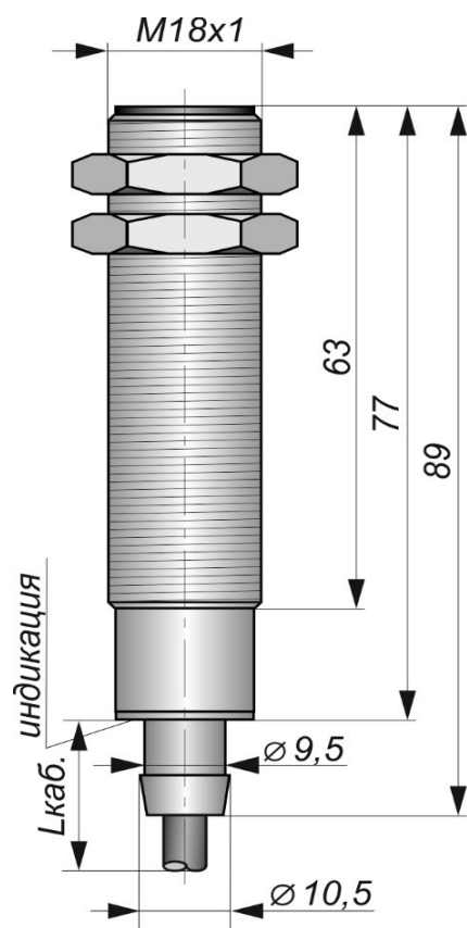
Габаритный чертеж
