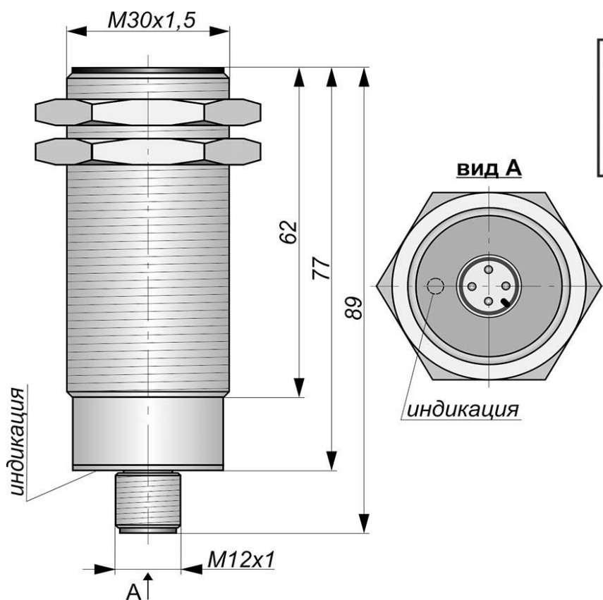
Габаритный чертеж
