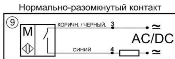
Схема соединения
