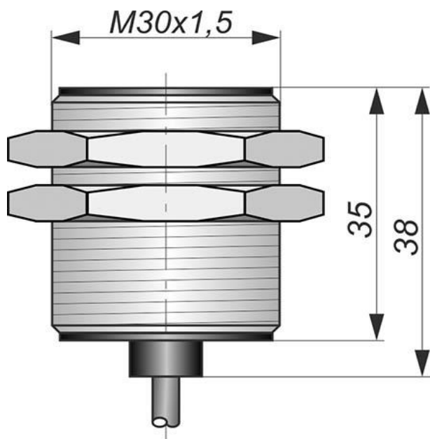
Габаритный чертеж
