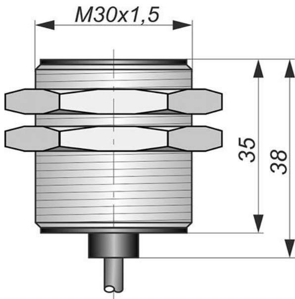
Габаритный чертеж
