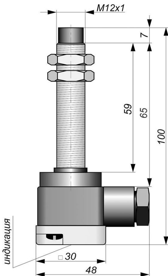
Габаритный чертеж
