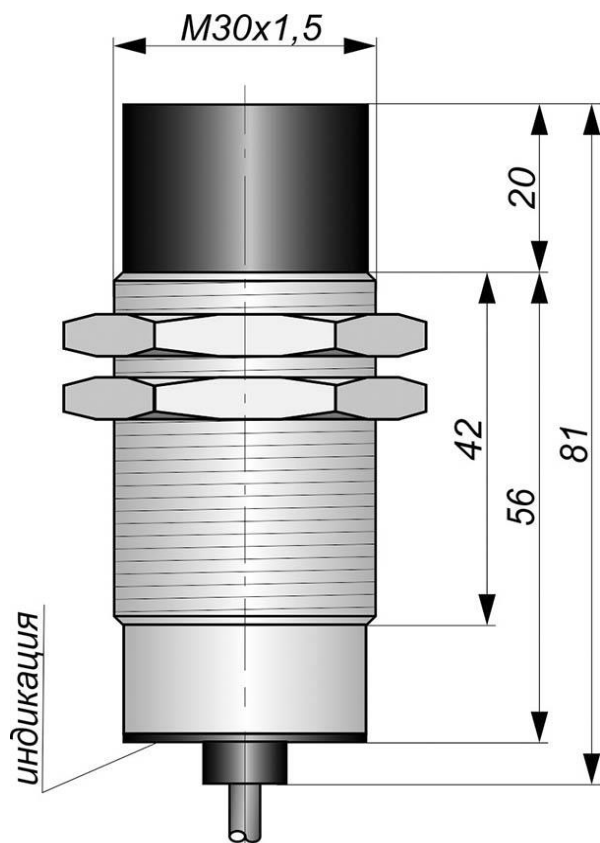
Габаритный чертеж
