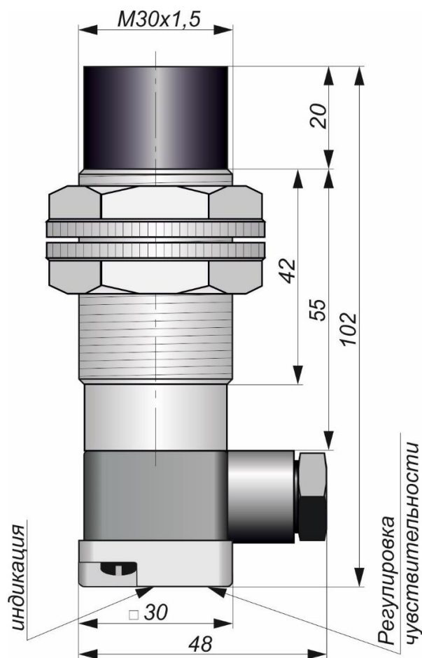
Габаритный чертеж
