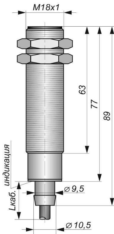
Габаритный чертеж
